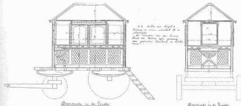
Doorsnede in de Lengte
